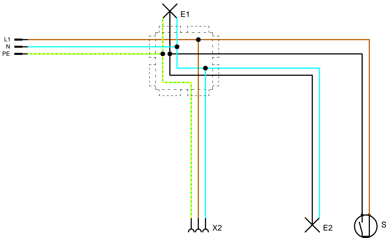
Bedradingschema
